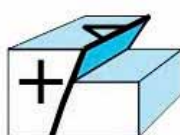
faglia verticale
